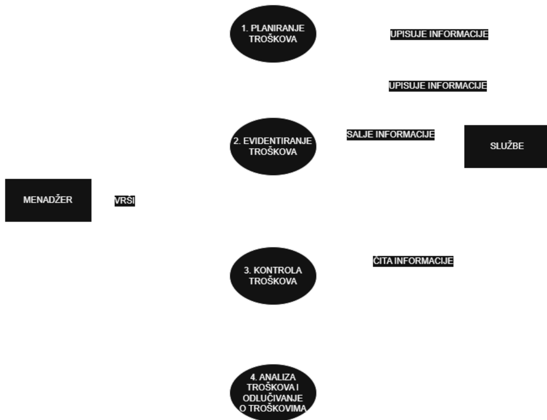
SSA prvi nivo dekompozicije
